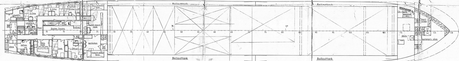
TWEEN DECK
